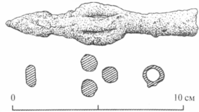
Наконечник болта от баллисты, обнаруженный при раскопках в Дура-Европос (Stephenson I. P. Roman Infantry Equipment. P. 96, 97)
