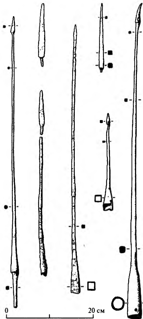
Пилумы первой половины III в. (Bishop M. C., Coulston J. C. N. Roman Military Equipment... P. 123)
