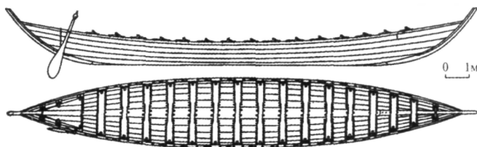
Англосаксонская барка. Конец IV в. ( Périn P., Feffer L. Ch. Les Francs. P. 41 )
