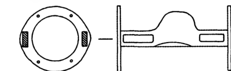
Натяжная рама от манубаллисты ( kambestria ). Найдена в Горнее (Румыния) ( Stephenson I. P. Roman Infantry Equipment. P. 94 )
