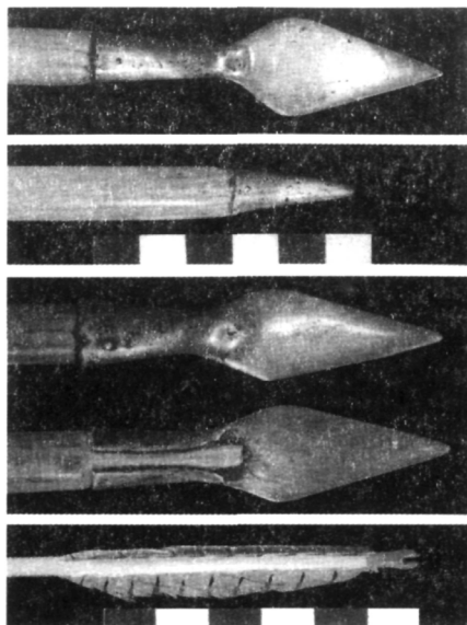
Различные типы наконечников стрел, использовавшихся в IV в. (Stephenson I. P. Roman Infantry Equipment. Colour plates 19–22)
