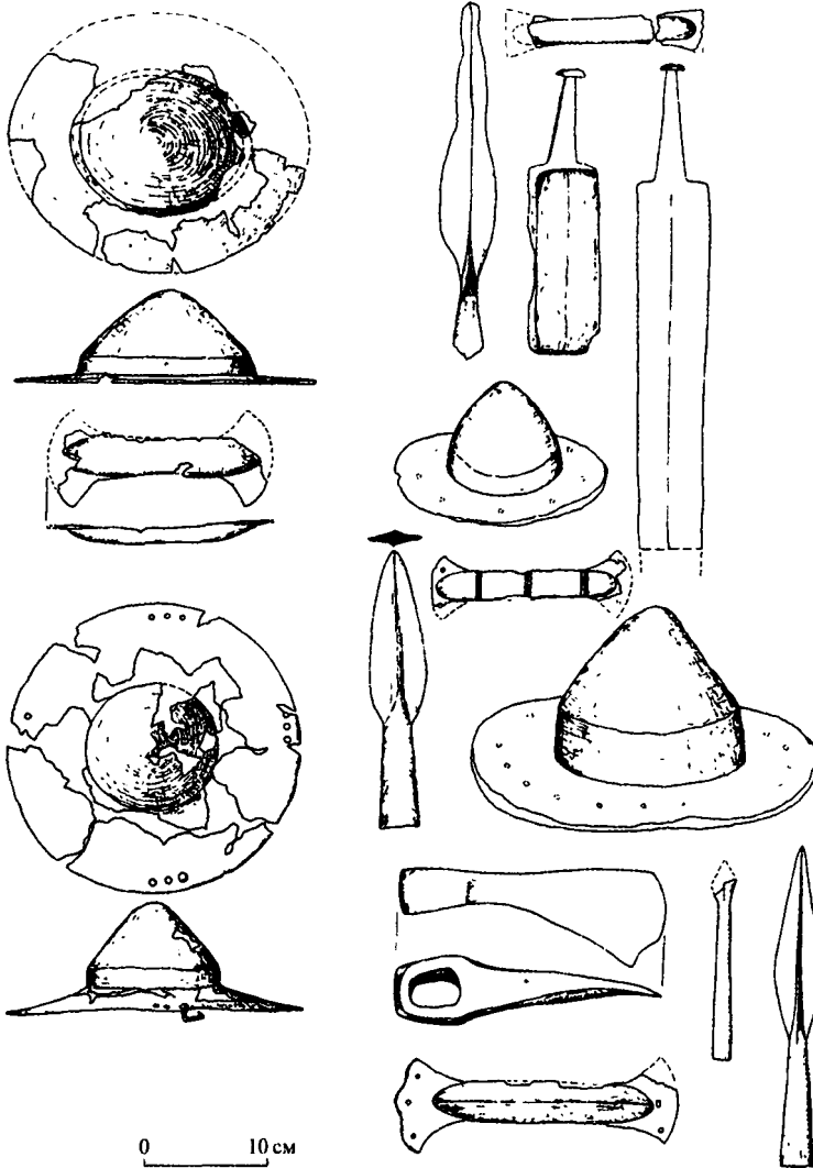
Готское оружие: умбоны и рукояти щитов, мечи, наконечники копий, лезвия секир (Kokowski A. L'art militaire des Goths... P. 348)
