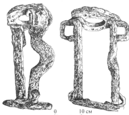
Две натяжные рамы ( kambestria ) от манубаллисты. Найдены в Орсове (Румыния) ( Stephenson I. P. Roman Infantry Equipment. P. 93 )
