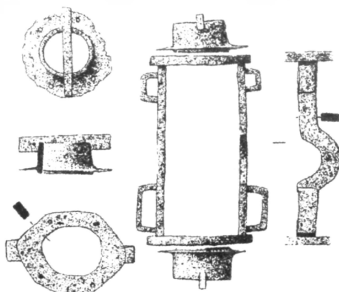
Натяжная рама ( kambestria ) и две втулки ( modioli ) от манубаллисты. Найдены в Лионе (Франция) ( Feugère M. Les armes... P. 218 )
