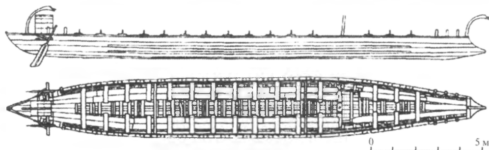
Реконструкция лусории из Майнца (тип А).
