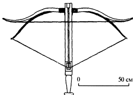
Реконструкция римского арбалета (Feugère M. Les armes... P. 214)
